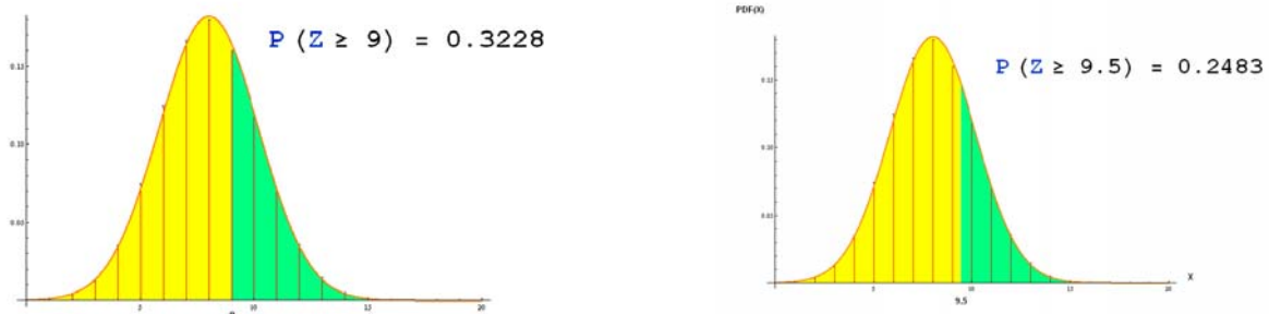
Figura 1.3: efecto de utilizar y = 9 o y = 9.5 sobre las probabilidades para calcular la aproximación de la normal a la binomial. La curva continua es la curva normal con la misma media y desviación típica que la binomial. Las líneas verticales representan la función de probabilidad de la binomial.
